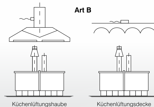
Küchenlüftungshaube
